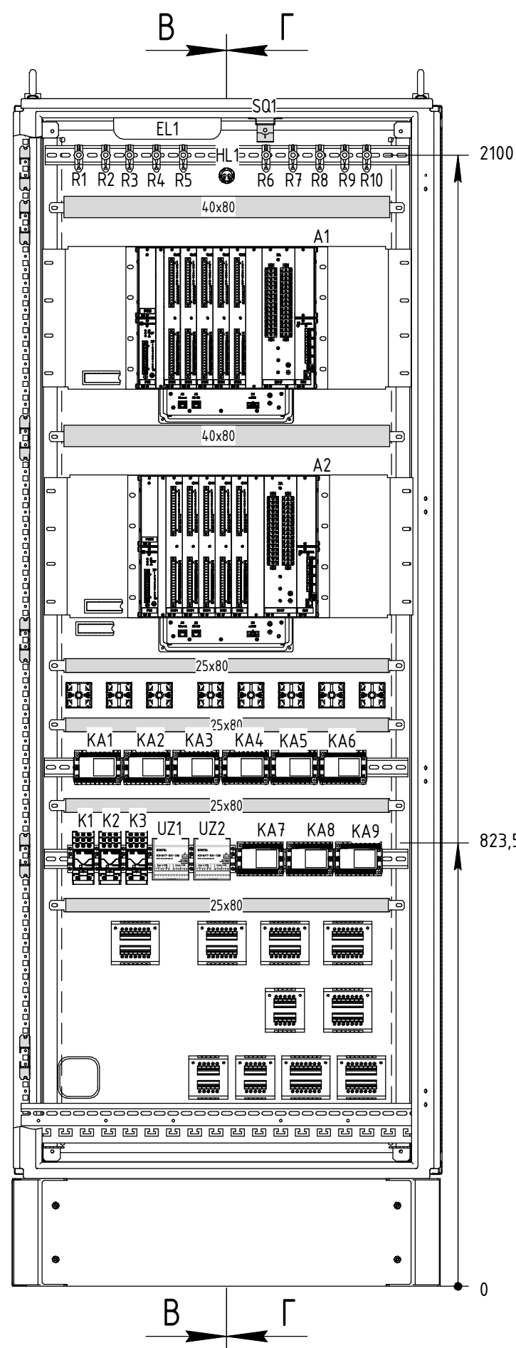
Вид сзади Дверь, ряды зажимов и вертикальные корпуса условно не показаны
