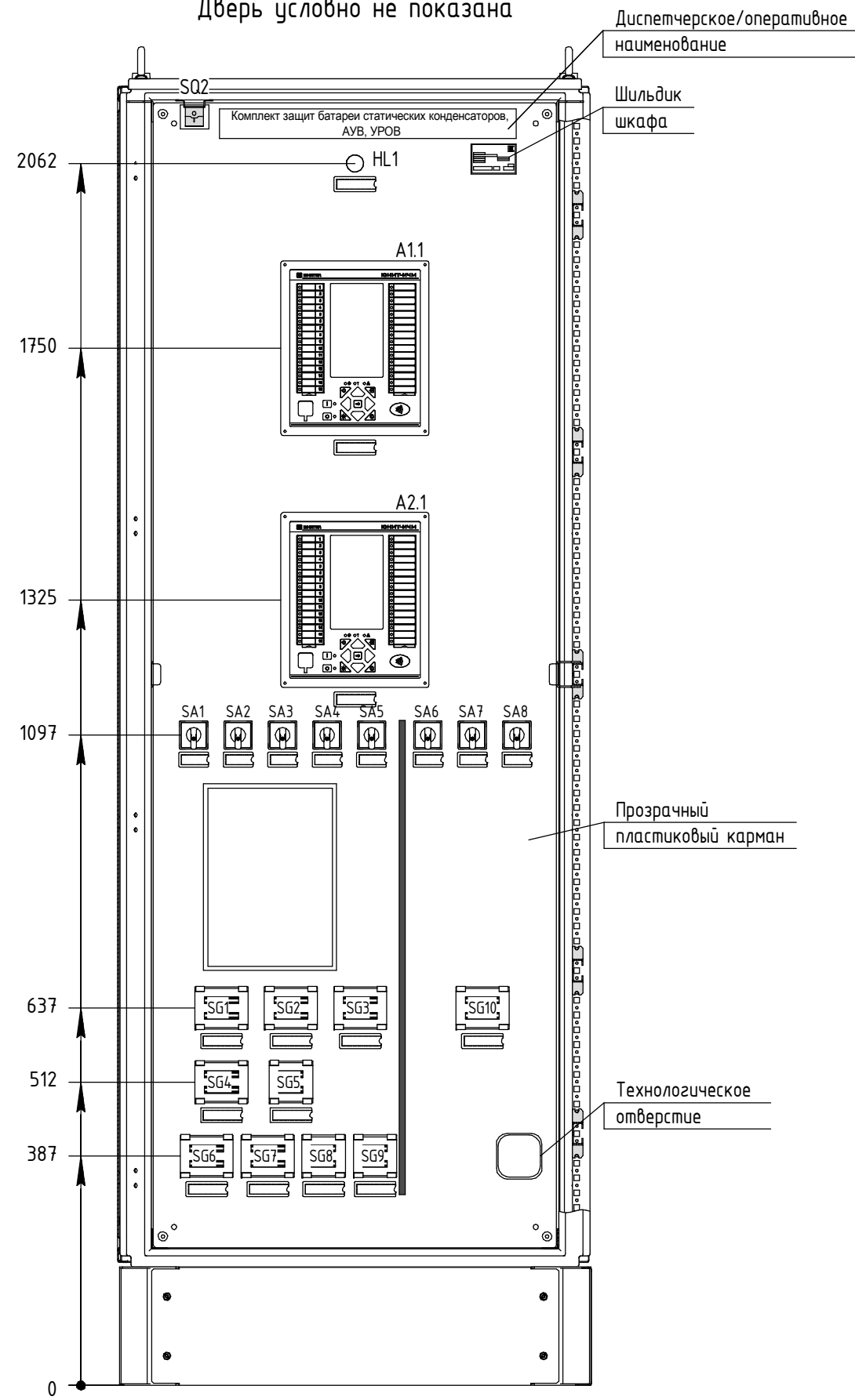
Вид спереди Дверь условно не показана
